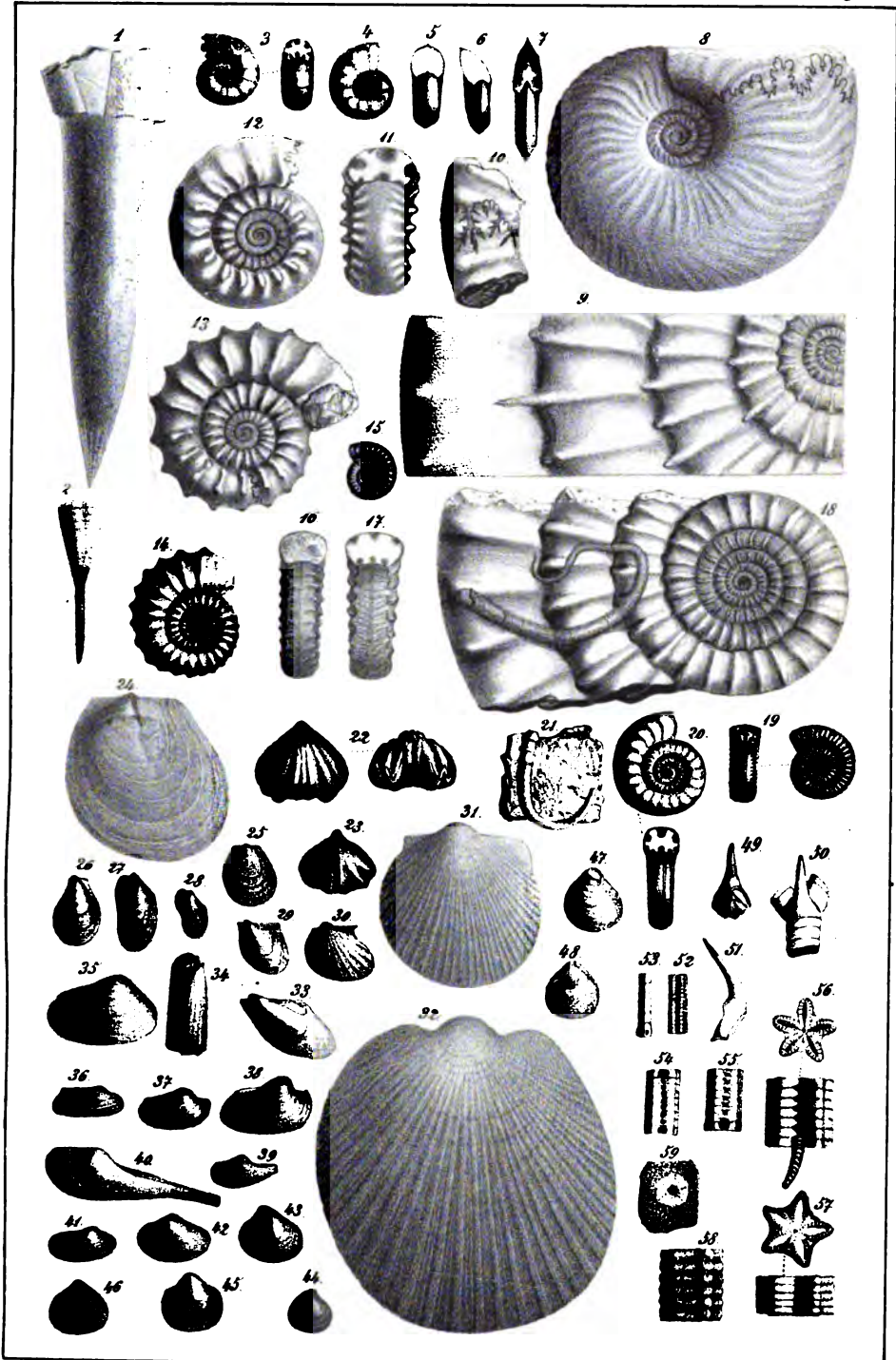
Quenstedt, Jura.
